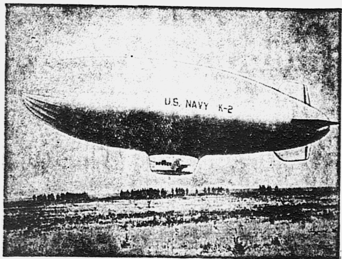
В США построен новый дирижабль «К-2». Это — один из крупнейших воздушных кораблей нежесткого типа. Его длина — 3,8 метр, объем — 401 тыс. куб. футов, он наполнен гелием. Гондола цельноалюминиевая, вмещает 8 человек. На снимке — дирижабль «К-2» поднимается с аэродрома в Акроне (штат Огайо). Расстояние около 800 км. дирижабль покрыл за 8 часов 25 минут. Фотохроника ТАСС.
